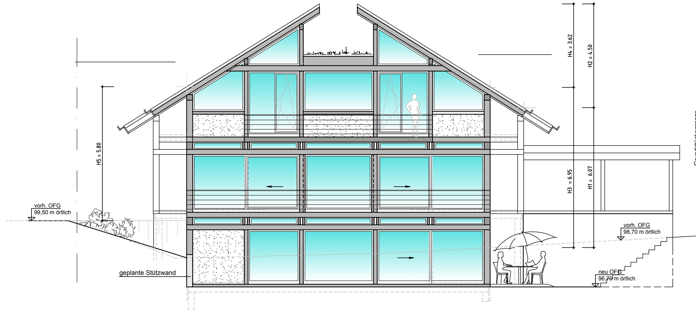
ANSICHT NORD - OST
