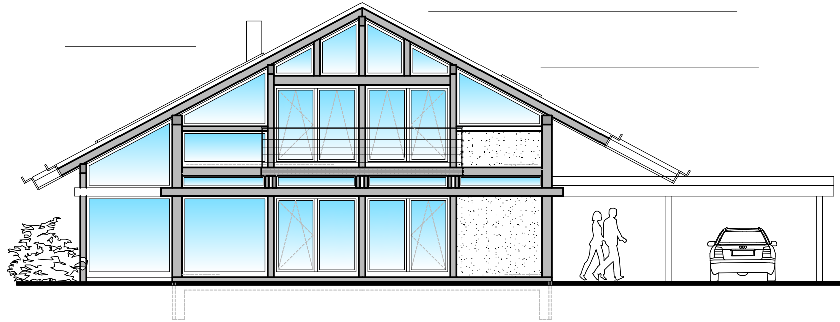
Ansicht Süd
